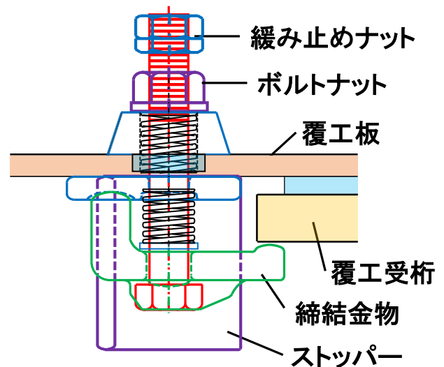
締結部拡大図
