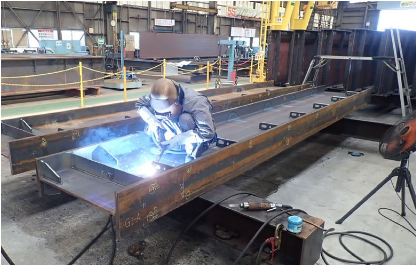
補剛材溶接
