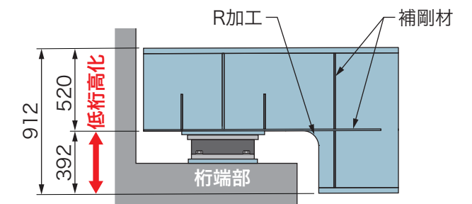
低桁高構造図
