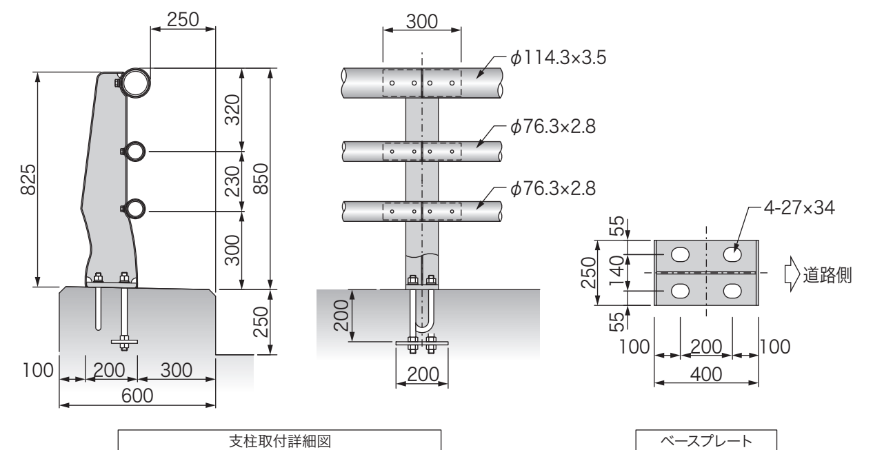
正面図
