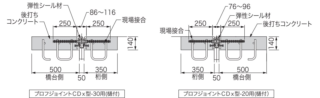
伸縮装置断面図（可動側）
