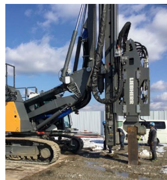
H鋼杭の打設状況
