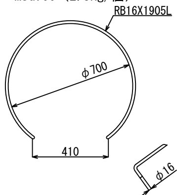
背当てガード MSG700 (2.3kg/個)
