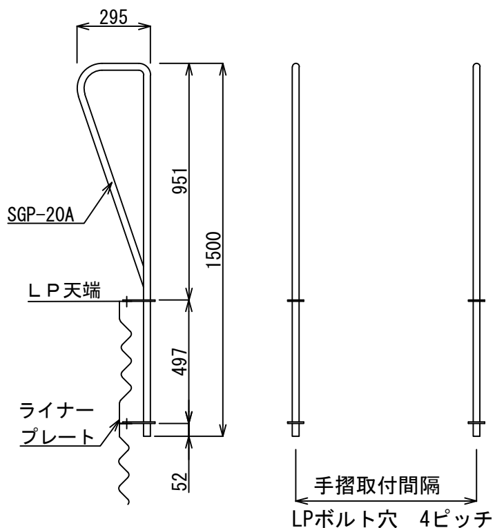
突き出し手摺り MTT1500 (4.8kg/個)
