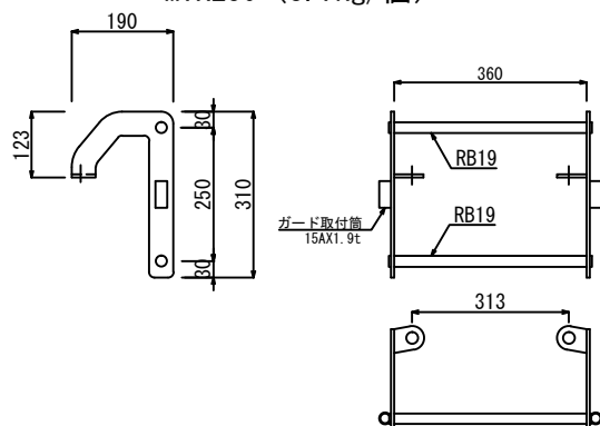
簡易タラップ MTR250 (3.7kg/個)
